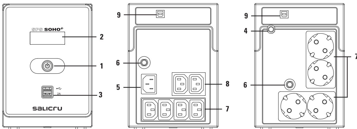
Fig. 2. Vista modelos SPS.SOHO+ 1200/1600VA.
